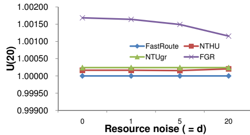
(d) U(20) variation
